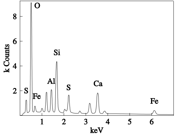
Fig. F- 3 EDS spectrum of point 2 – ettringite
