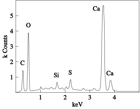
Fig. F- 5 EDS spectrum of point 4 – ettringite
