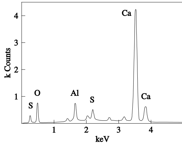
Fig. F- 7 EDS spectrum of point 6 - ettringite
