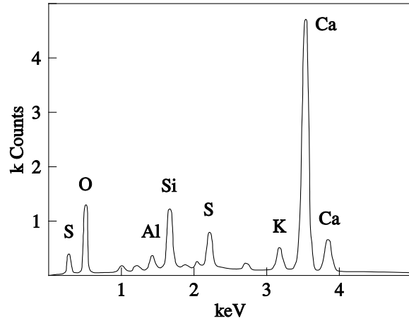
Fig. F- 6 EDS spectrum of point 5 – ettringite
